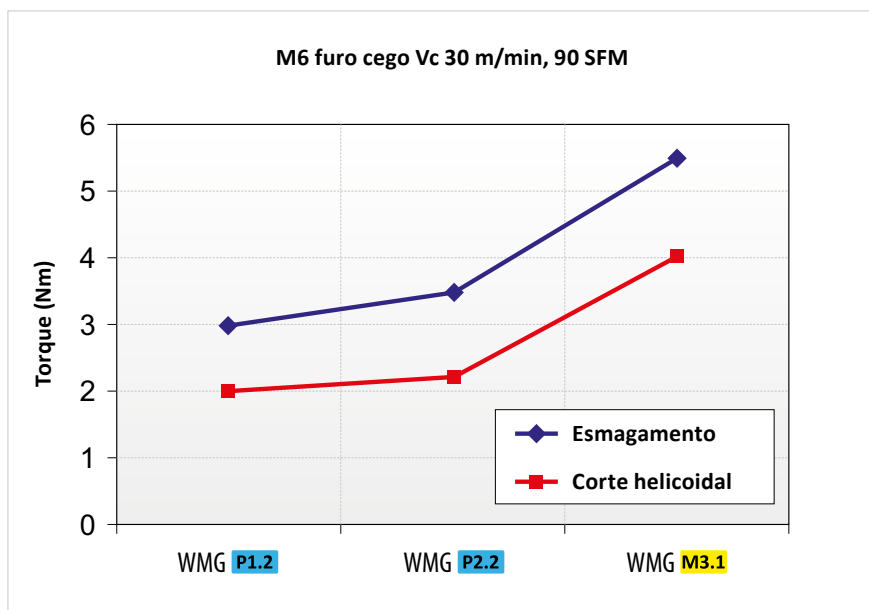
Comparação de torque entre machos de esmagamento e de corte em diferentes grupos de materiais.
